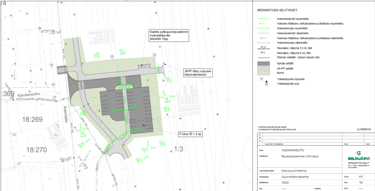
Kuva 17 Luonnosvaiheen suunnitelma pysäköintialueesta
