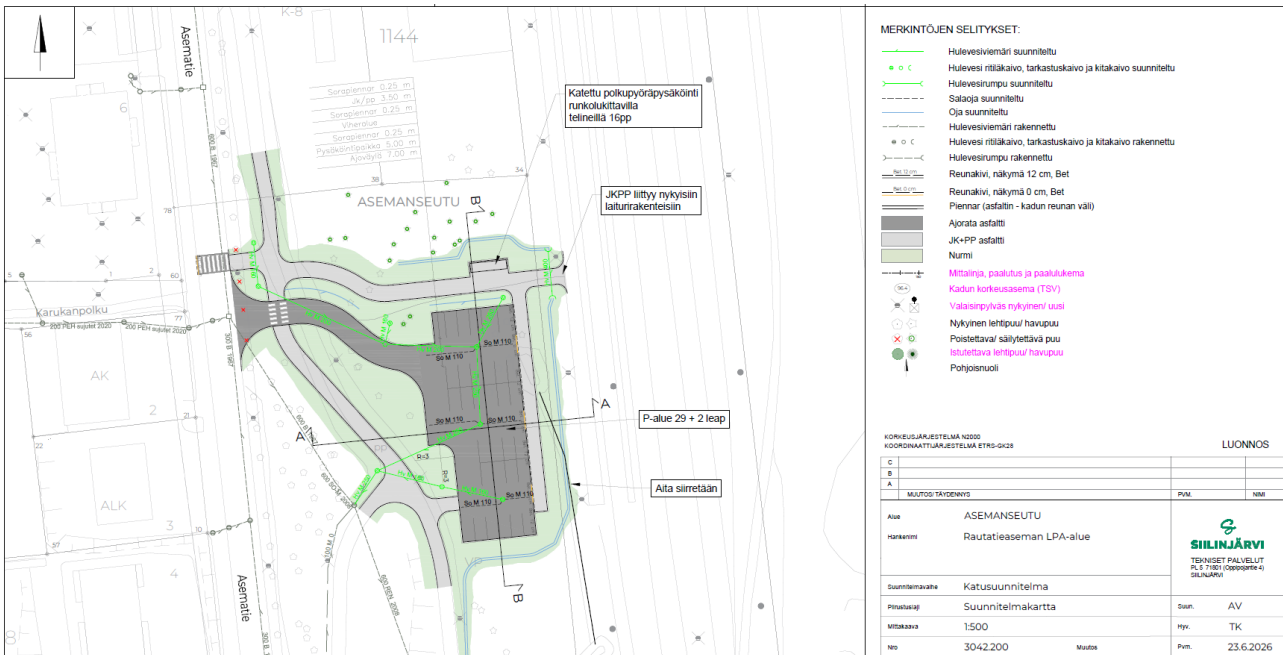
Kuva 18 Ehdotusvaiheen päivitetty suunnitelma pysäköintialueesta
