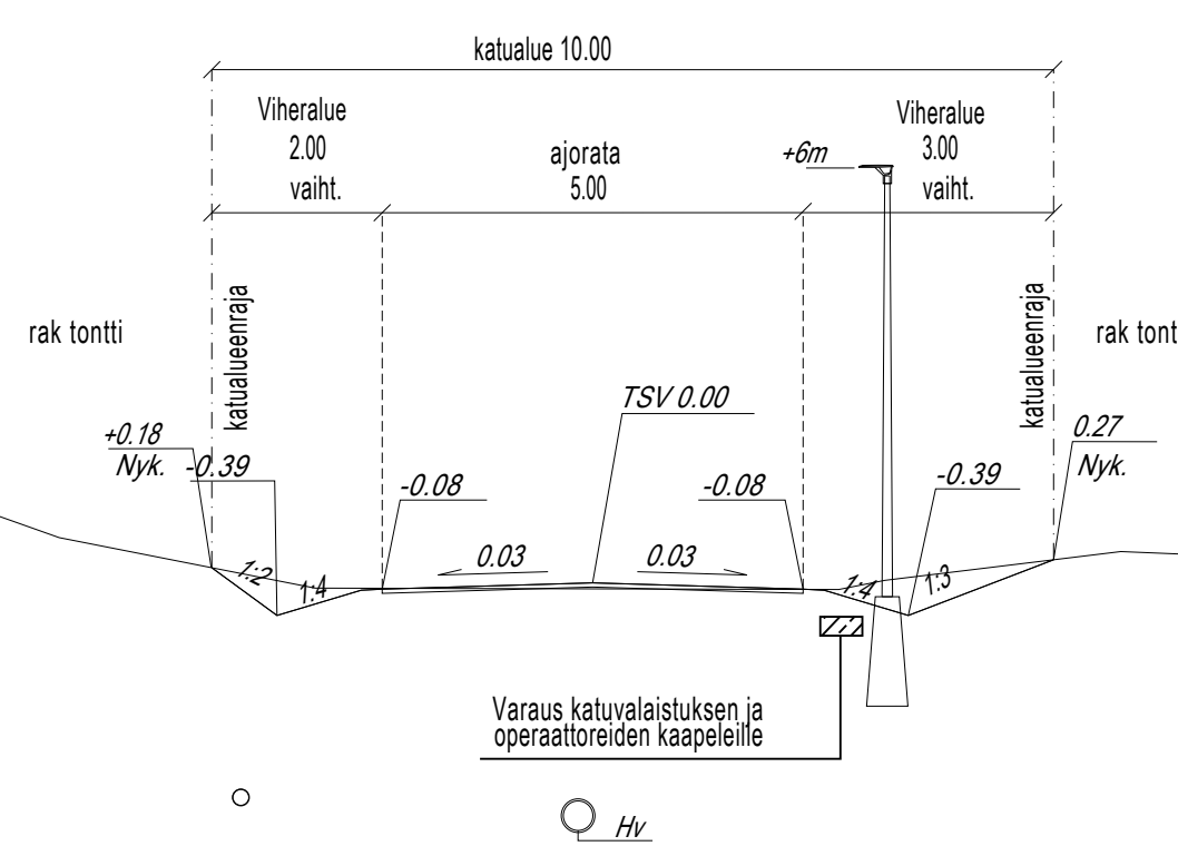
Huhtakierto pl 50 Tyyppipoikkileikkaus A-A
