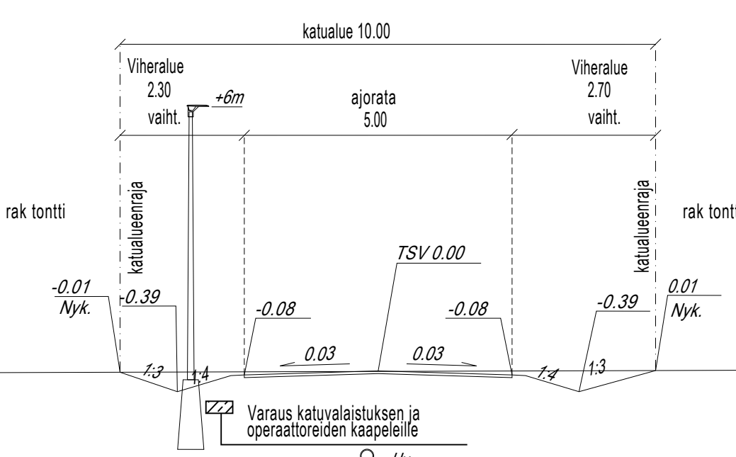
Kaskipolku pl 70 Tyyppipoikkileikkaus A-A
