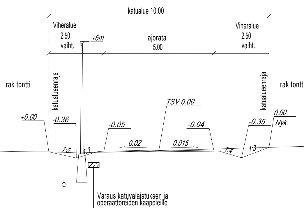
Kirvespolku pl 20 Tyyppipoikkileikkaus A-A
