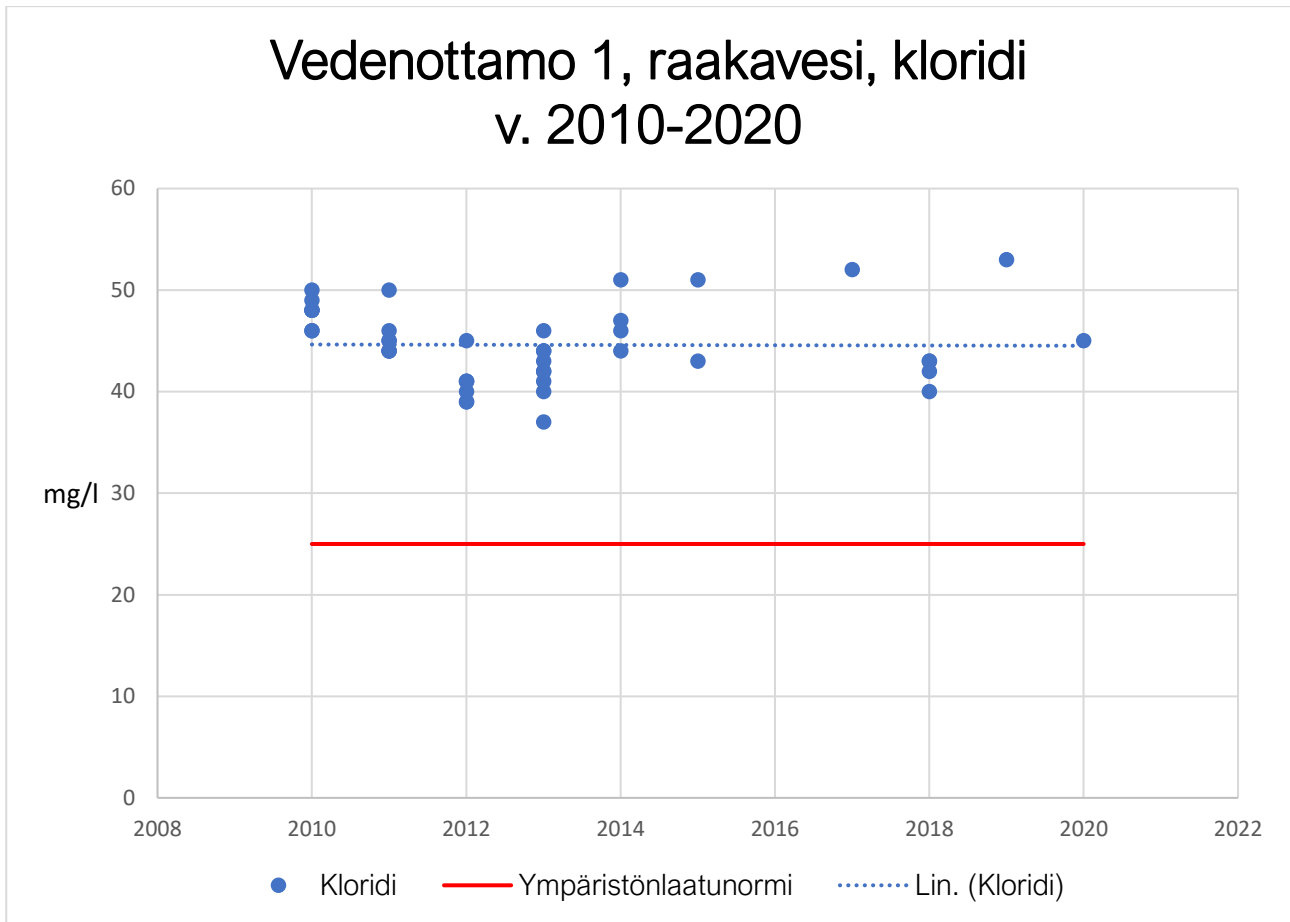
Kuva 6. Vedenottamo 1, raakaveden kloridipitoisuus v. 2010–2020
